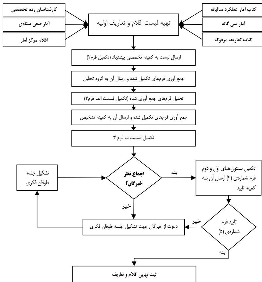
شکل شماره ۱: فلوچارت استاندارد سازی تعاریف و اقدام آماری ناجا
